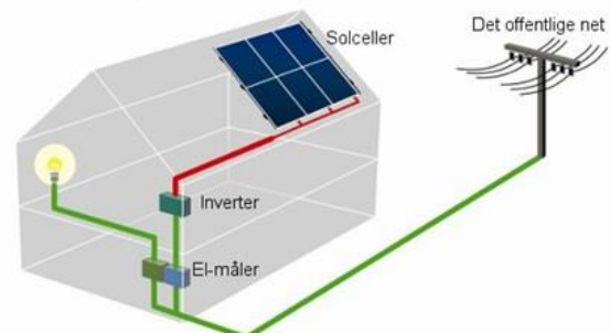
Principskitse af et solcelleanlæg
